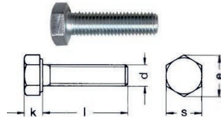
DIN933 - VOLLGEWINDE
