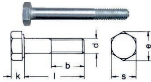
DIN931 - TEILGEWINDE
